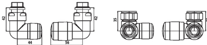
Комплект малогабаритных запорно-регулирующих вентилей - Рис. 7
