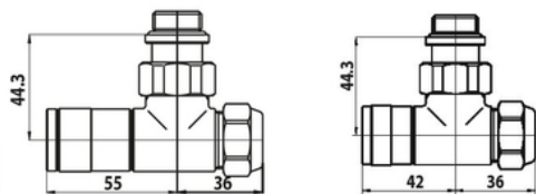
Комплект запорно-регулирующих вентилей для углового подключения - Рис. 5
