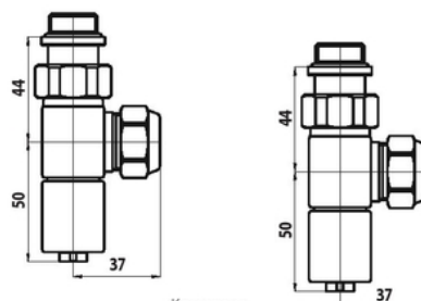
Комплект запорно-регулирующих вентилей - Рис. 6
