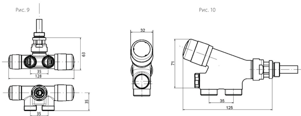
Комплект с термостатическим вентилем для углового однотрубного подключения (Рис. 9)
